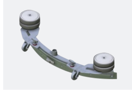
4 Stötfångare för höga hjul för gummiskrapa
