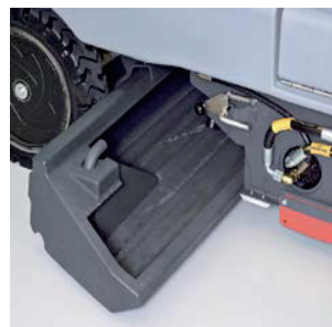
42L スライド式ホッパー
